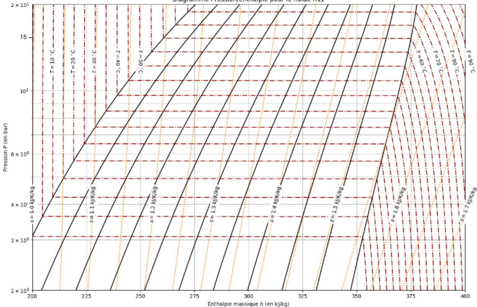
Diagramme Pression/Enthalpie pour le fluide R12
