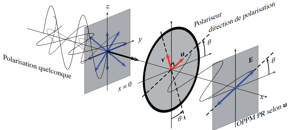
FIGURE 19 – Fonctionnement d'un polaroïd utilisé en polariseur
