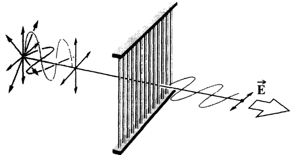
FIGURE 20 – Polariseur à grille
