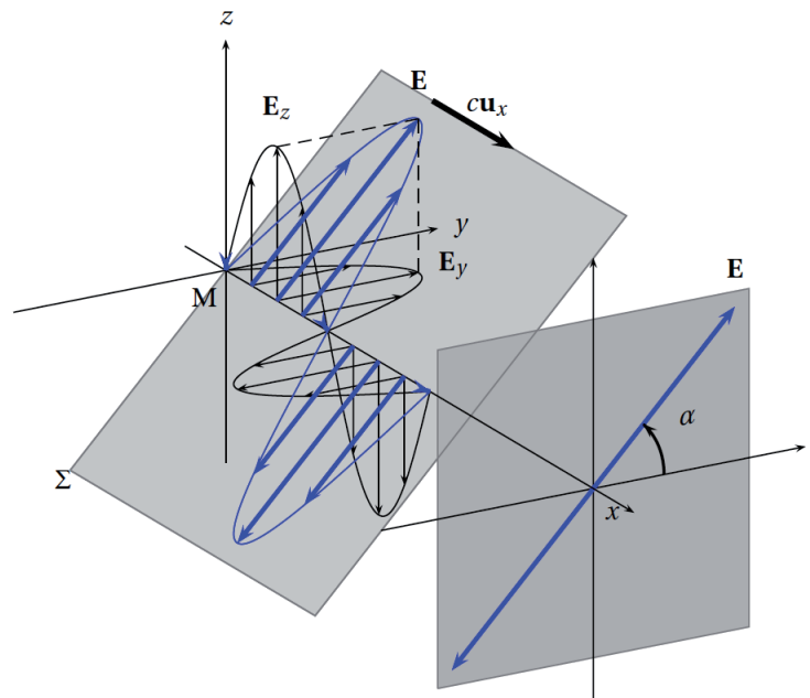
FIGURE 7 – O.P.P.H. électrique polarisée rectilignement
