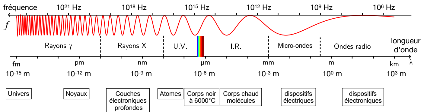
FIGURE 1 – Spectre électromagnétique
