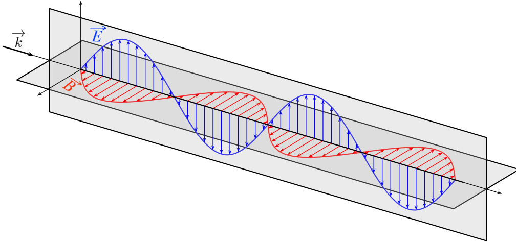
FIGURE 6 – Propagation d'une O.P.P.H.
