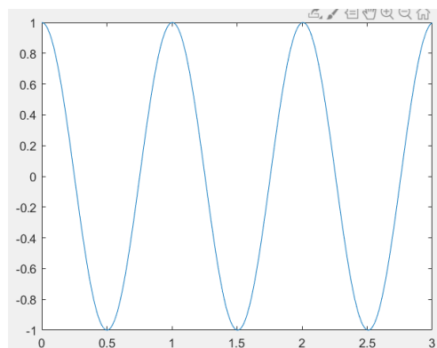
RUNGE KUTTA
